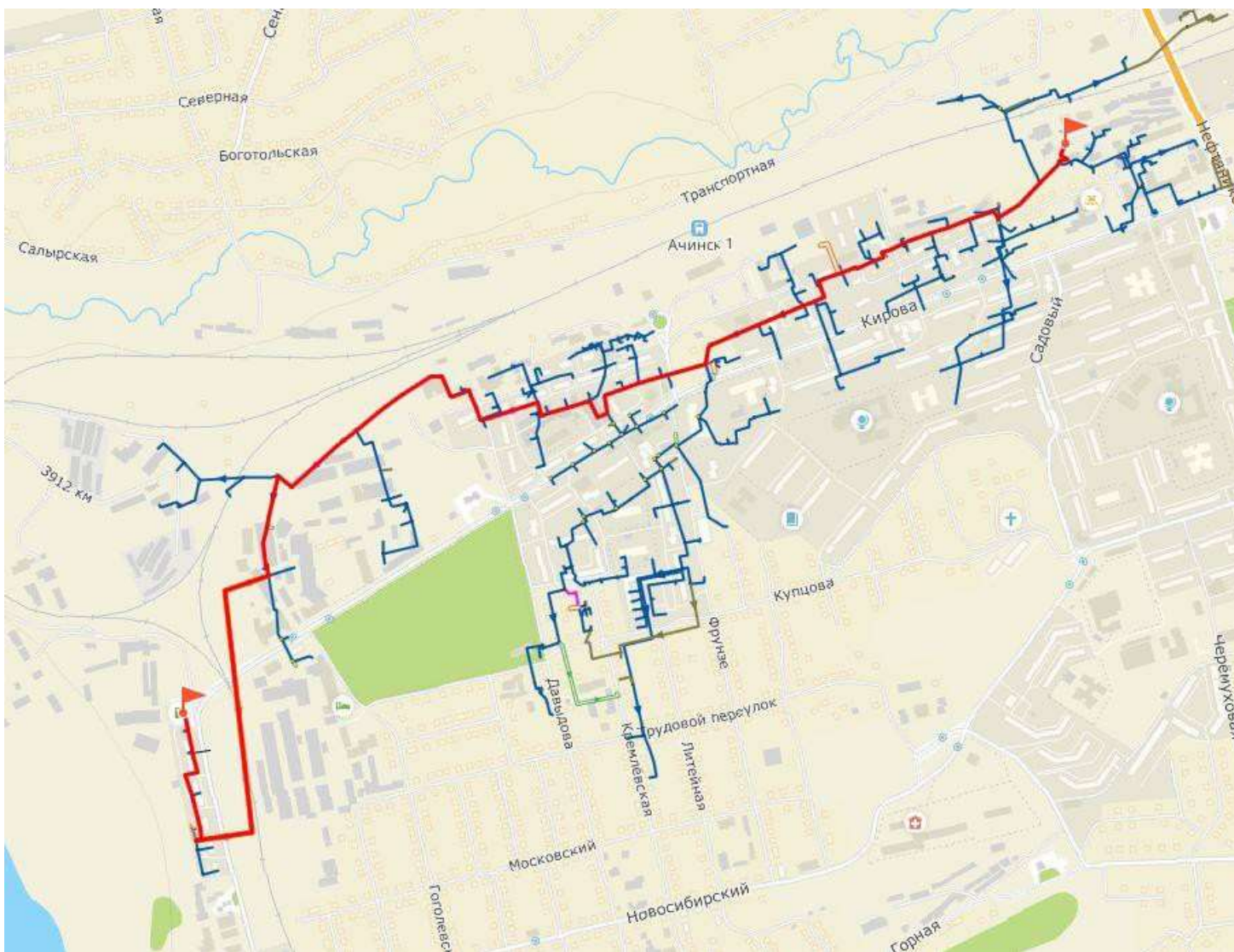
Рисунок 4.2.19. Путь построения пьезометрического графика котельная №6 – АЗС
