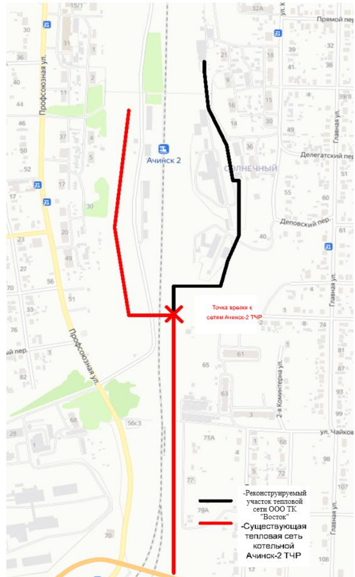
Рисунок 4.2.6. Перспективная схема сетей котельной ОАО «РЖД»
