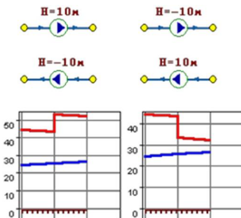
Рисунок 3.2.15. Пьезометрические графики
