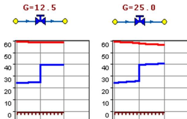
Рисунок 3.2.20. Регулятор давления
