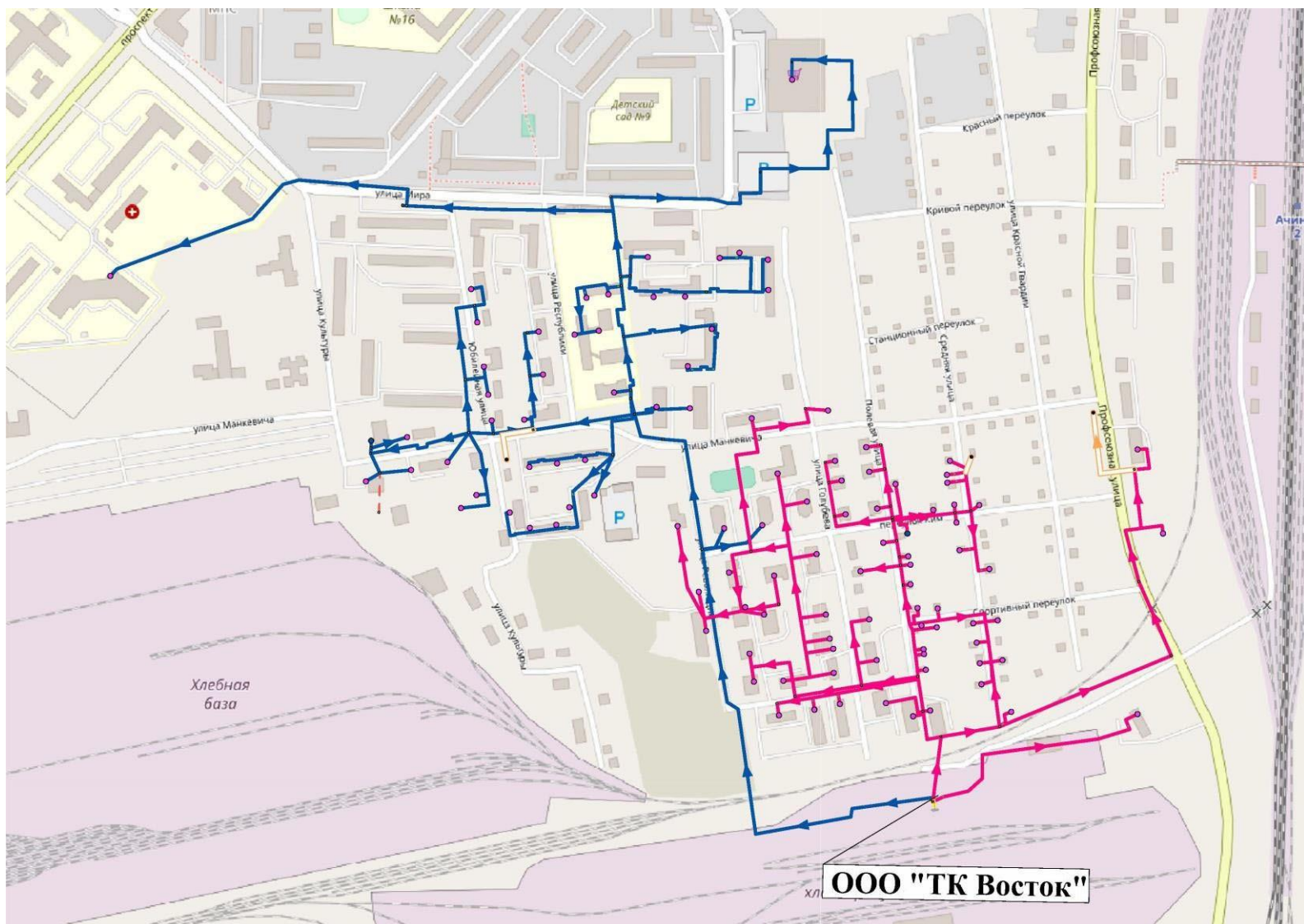
Рисунок 4.2.5. Перспективная схема сетей котельной ООО «ТК Восток»
