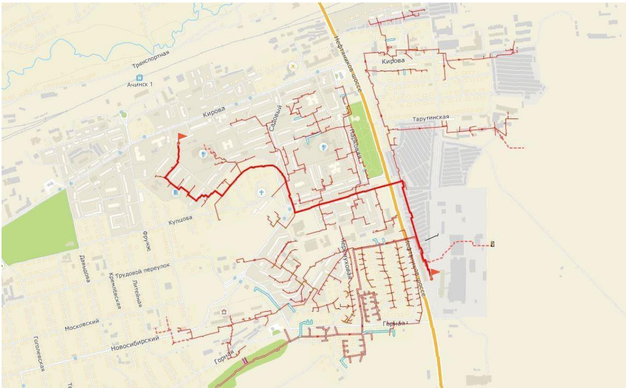
Рисунок 1.3.8.7 - Путь пьезометрического графика от ЦТП до Кирова, 41
