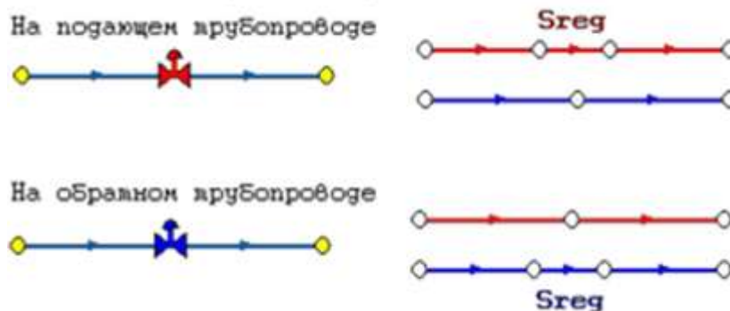
Рисунок 3.2.17. Дросселирующие устройства
