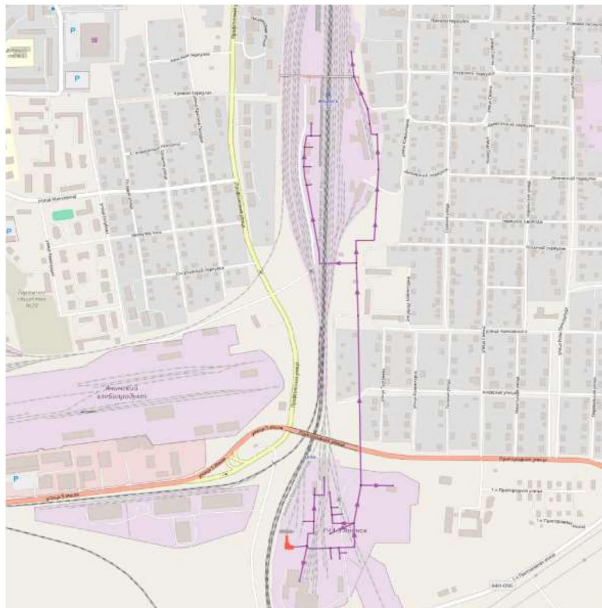
Рисунок 4.2.6. Перспективная схема сетей котельной ОАО «РЖД»
