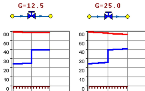
Рисунок 3.2.20. Регулятор давления
