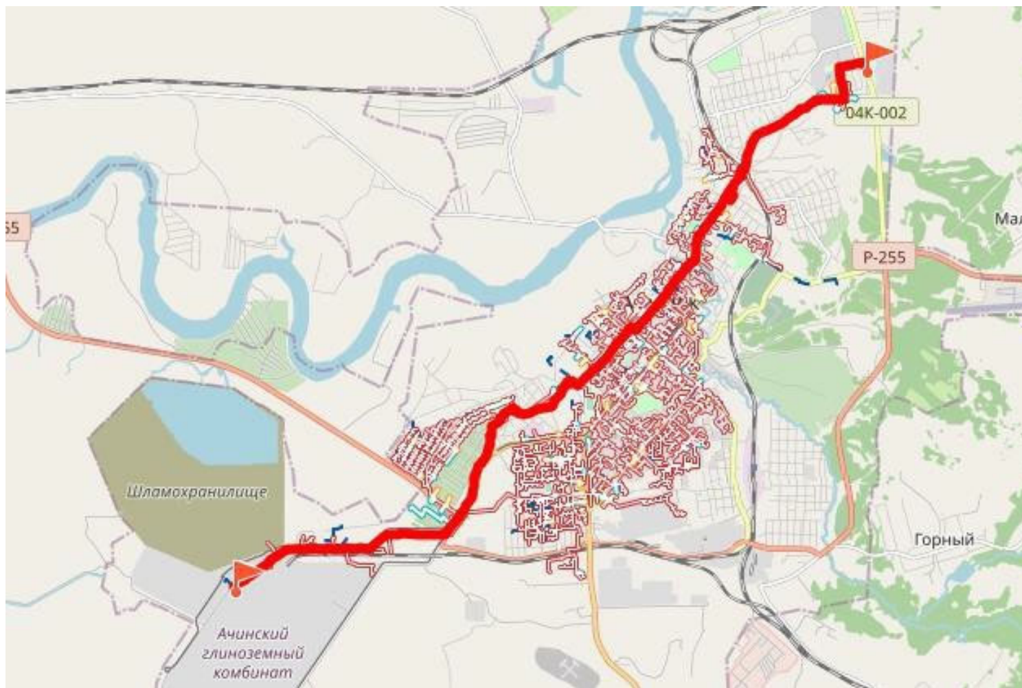
Рисунок 4.2.11. Путь построения пьезометрического графика ТЭС АО «РУСАЛ Ачинск» – ЦТП
